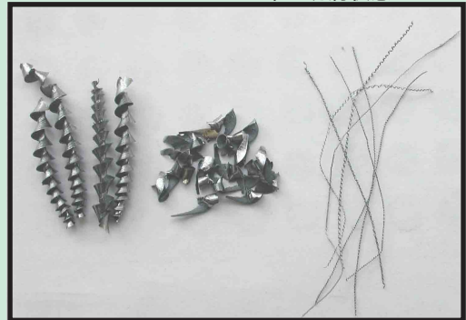
MEGAドリルリーマーの正常な切屑状態
